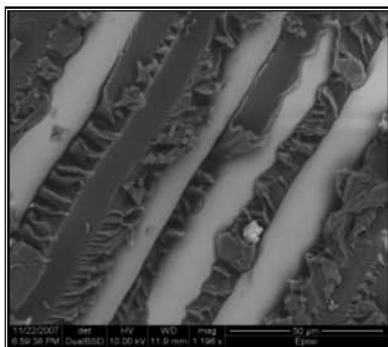
GV (UD)-Epoxy laminate
